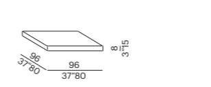
piano tavolo basso - top for low table 96
