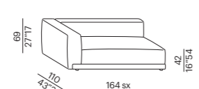
elemento angolo - corner unit 165
