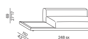
elemento con tavolo basso - unit with low table 250
